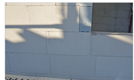
Nicht eingehaltenes Versatzmaß – Rissbildungsgefahr im Putz.
